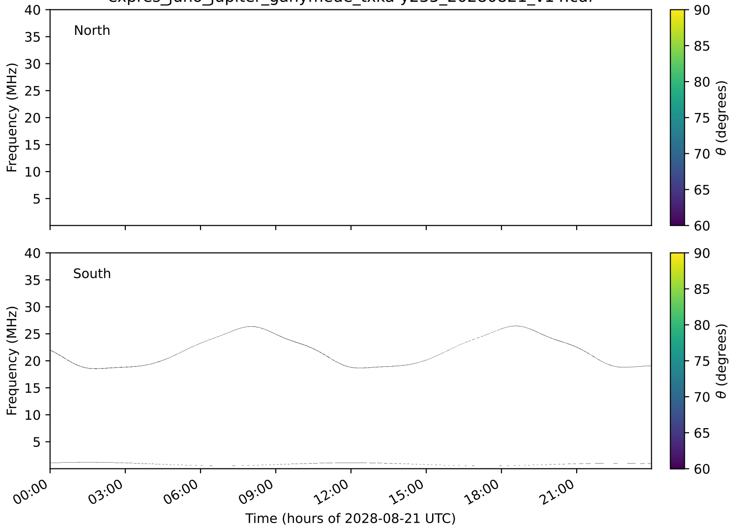
expres_juno_jupiter_ganymede_txka-y235_20280821_v14.cdf
