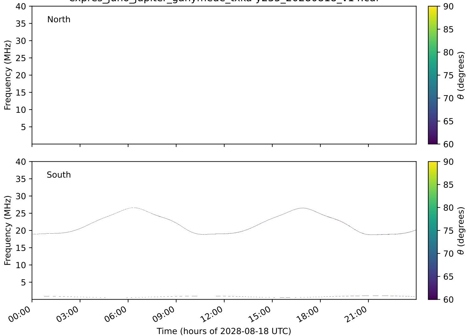
expres_juno_jupiter_ganymede_txka-y235_20280818_v14.cdf
