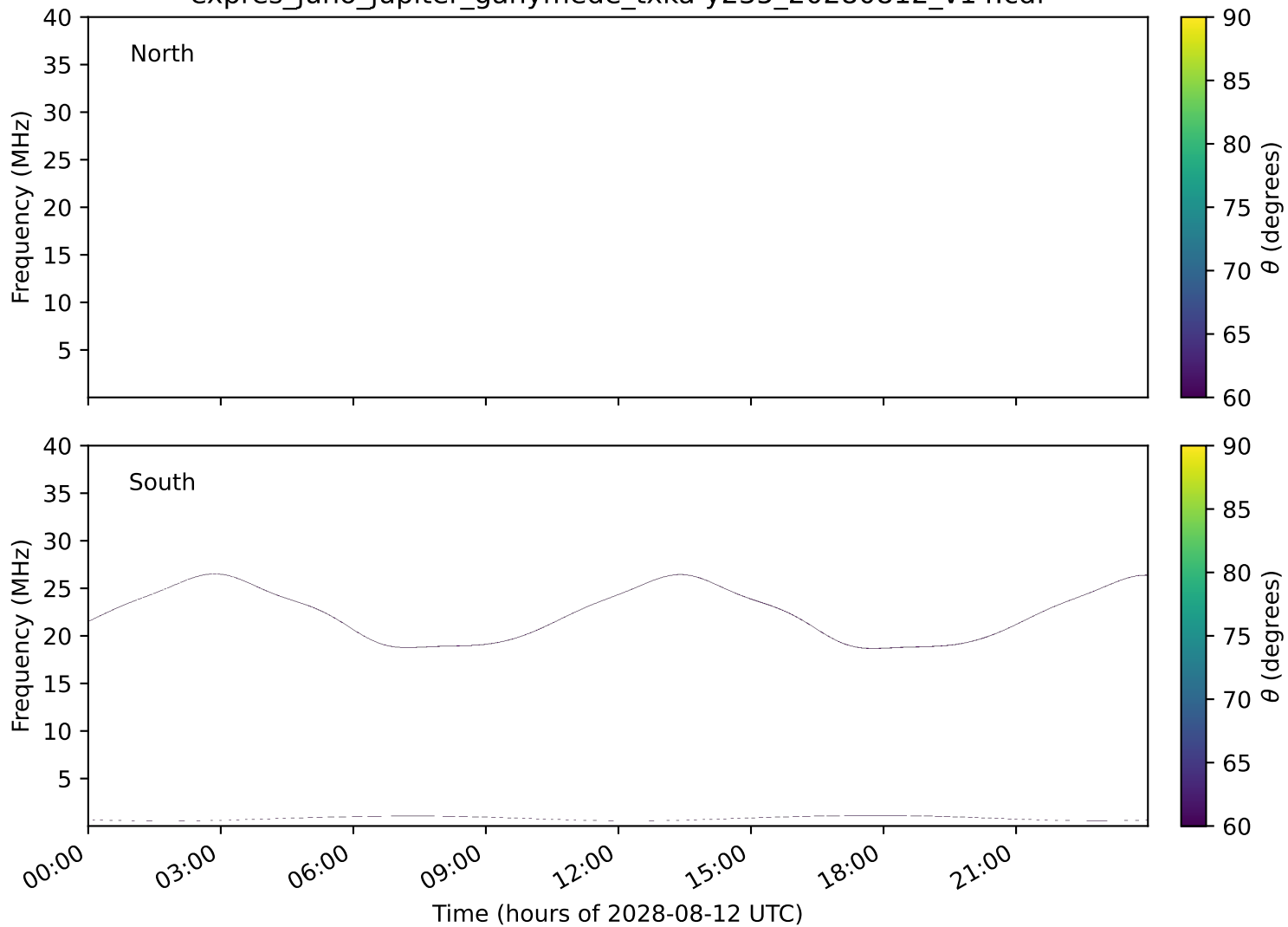
expres_juno_jupiter_ganymede_txka-y235_20280812_v14.cdf
