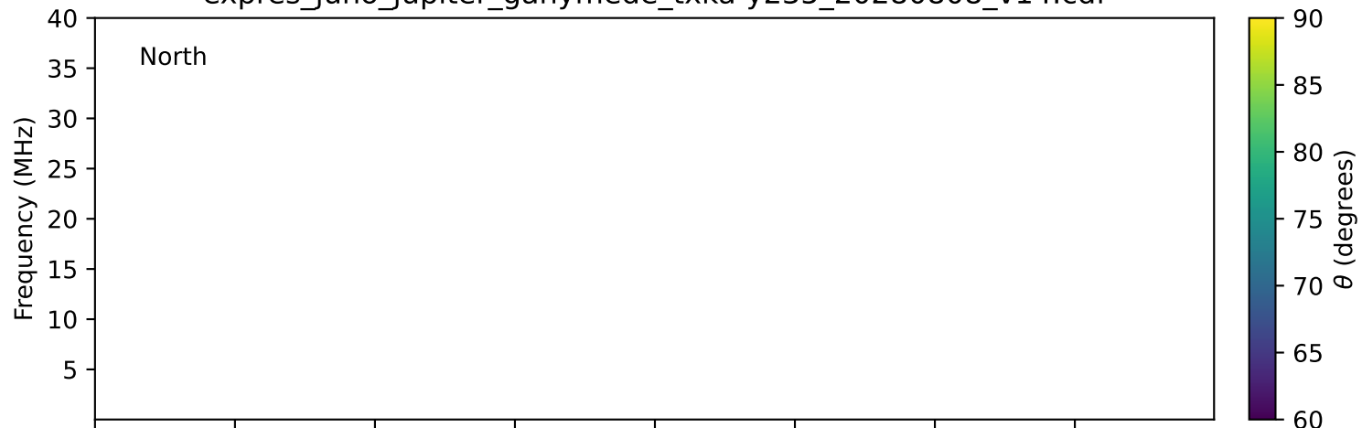
expres_juno_jupiter_ganymede_txka-y235_20280808_v14.cdf
