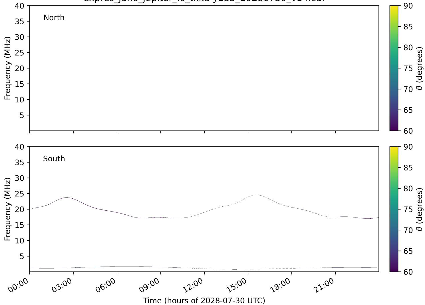
expres_juno_jupiter_io_txka-y235_20280730_v14.cdf
