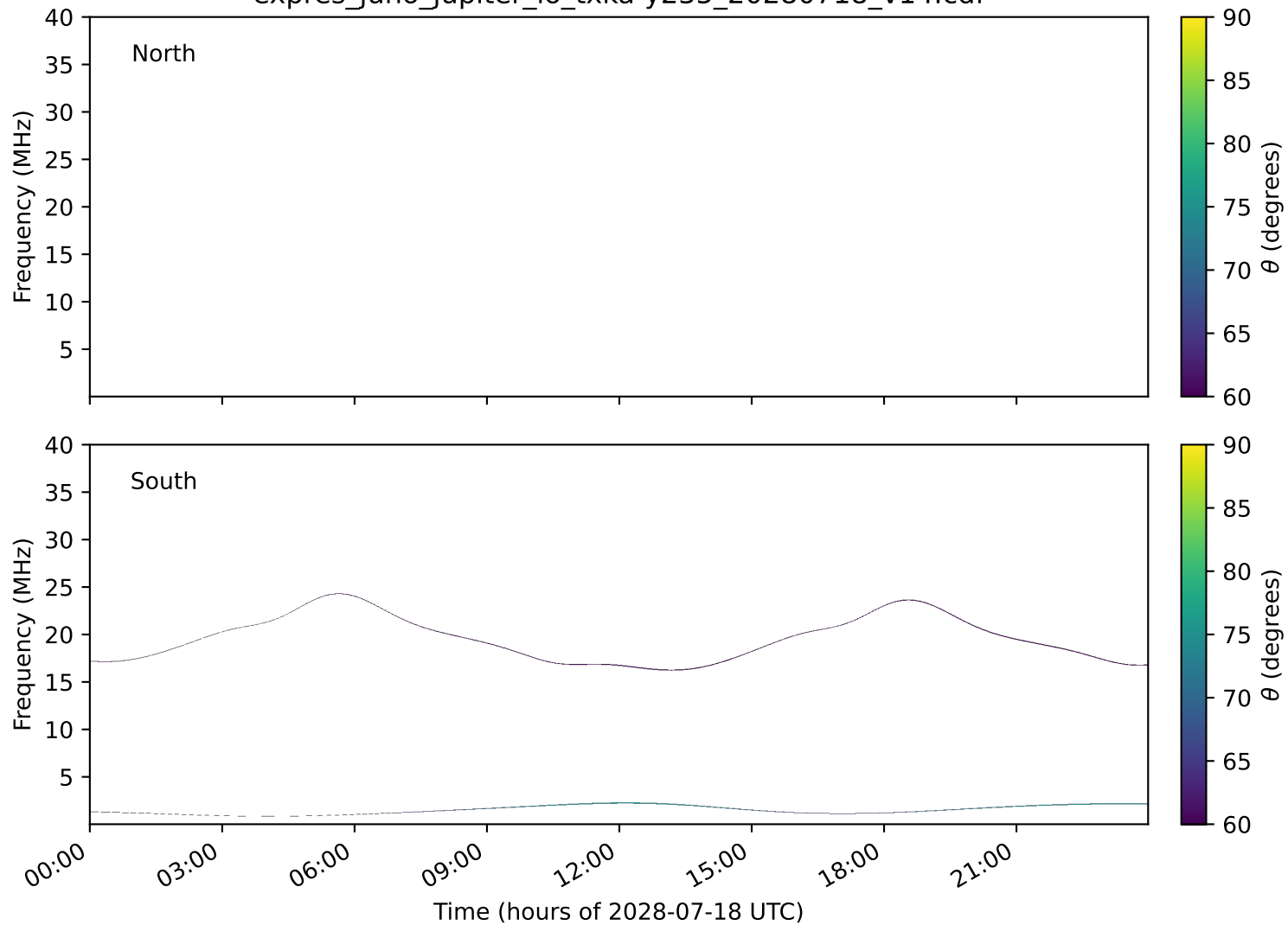
expres_juno_jupiter_io_txka-y235_20280718_v14.cdf
