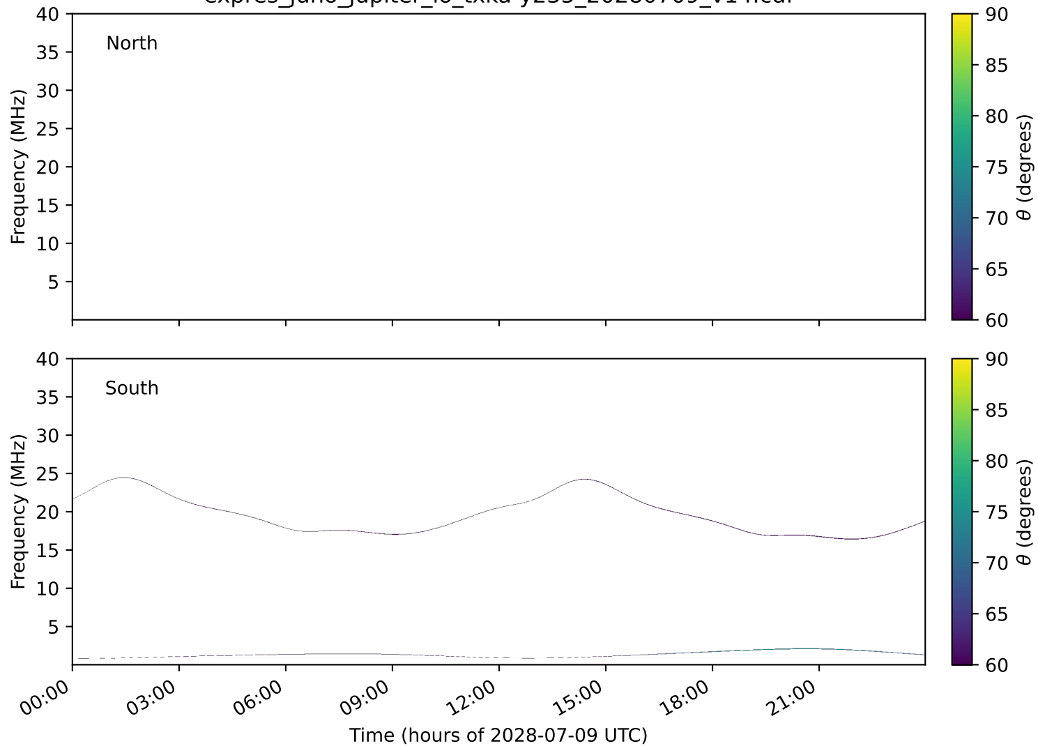
expres_juno_jupiter_io_txka-y235_20280709_v14.cdf
