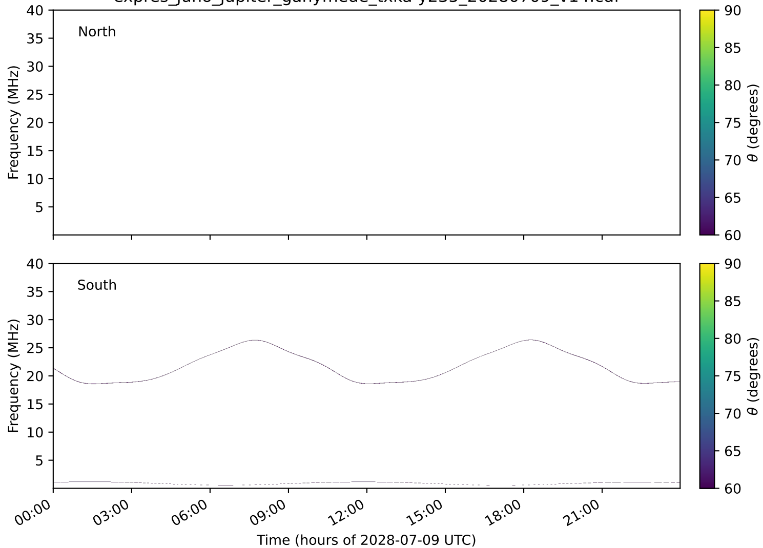
expres_juno_jupiter_ganymede_txka-y235_20280709_v14.cdf
