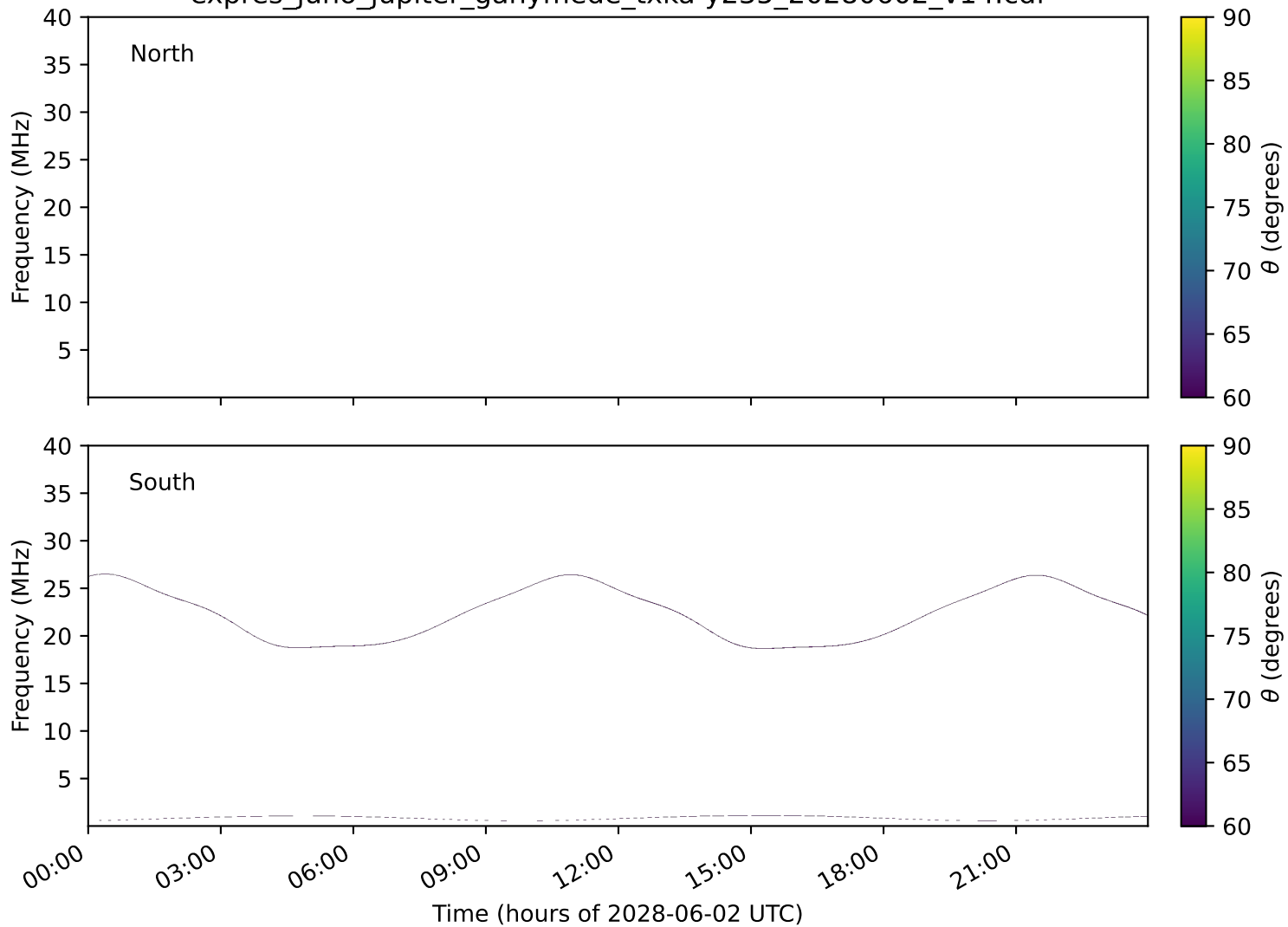
expres_juno_jupiter_ganymede_txka-y235_20280602_v14.cdf
