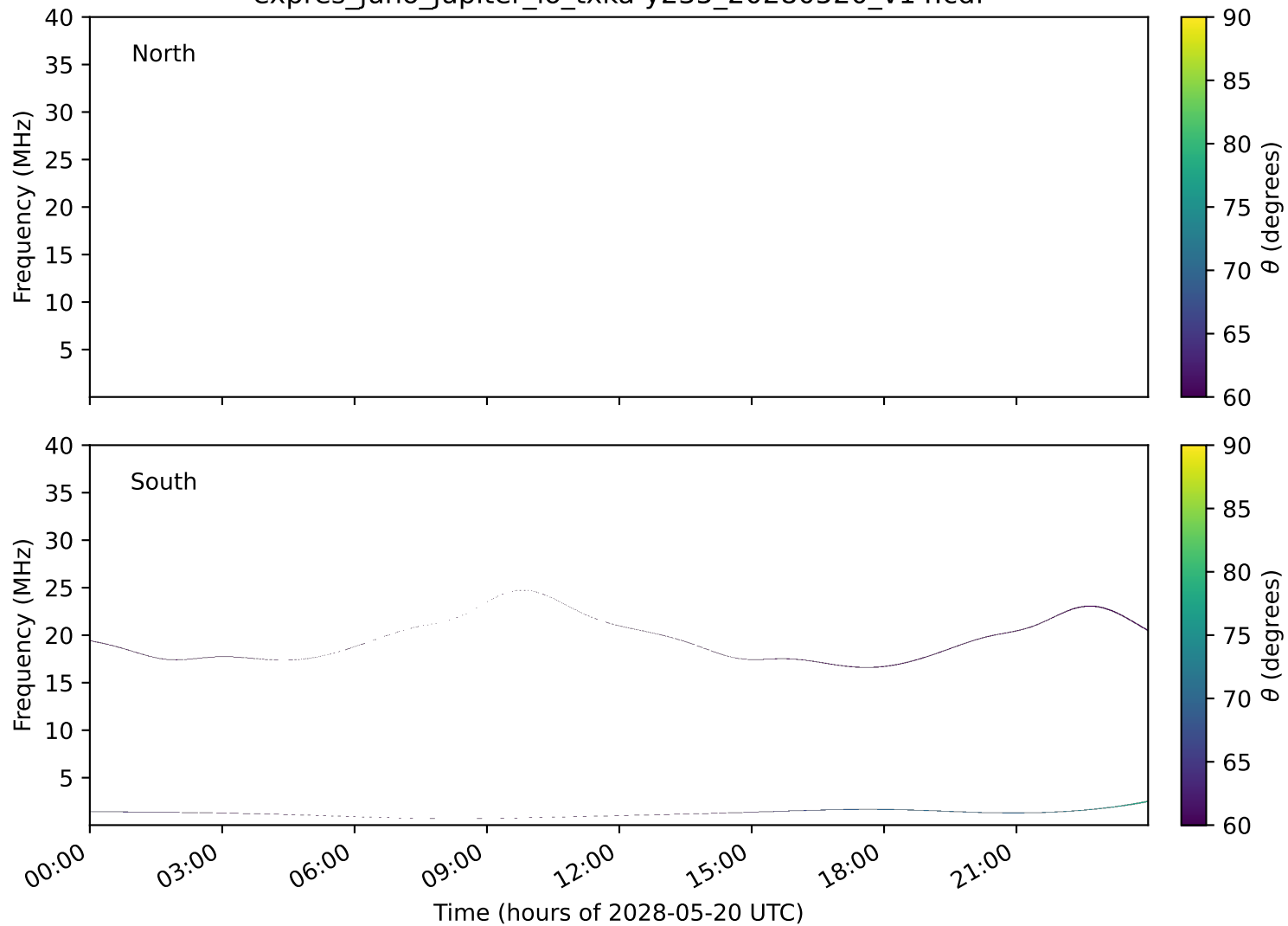
expres_juno_jupiter_io_txka-y235_20280520_v14.cdf
