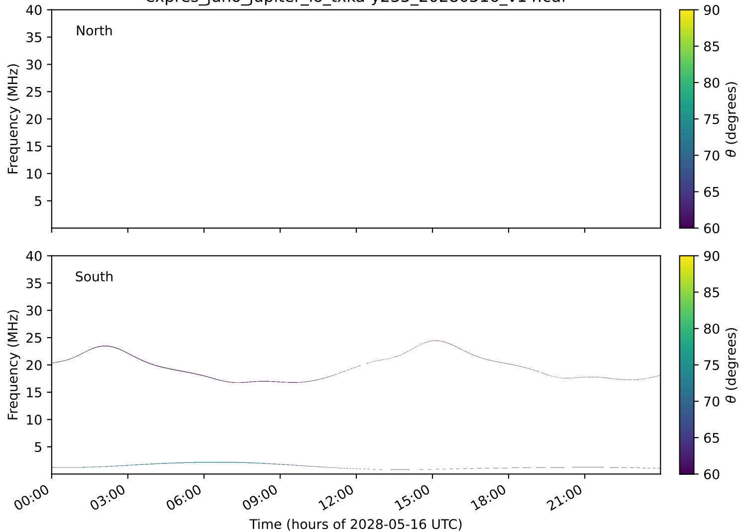
expres_juno_jupiter_io_txka-y235_20280516_v14.cdf
