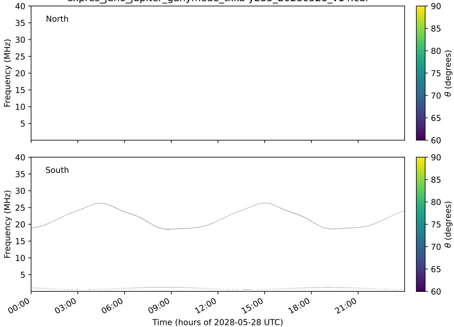
expres_juno_jupiter_ganymede_txka-y235_20280528_v14.cdf
