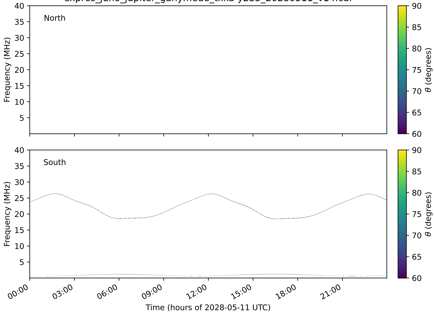
expres_juno_jupiter_ganymede_txka-y235_20280511_v14.cdf
