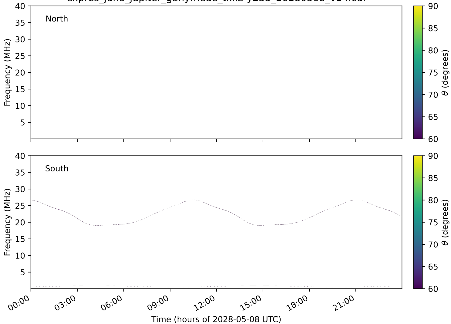
expres_juno_jupiter_ganymede_txka-y235_20280508_v14.cdf
