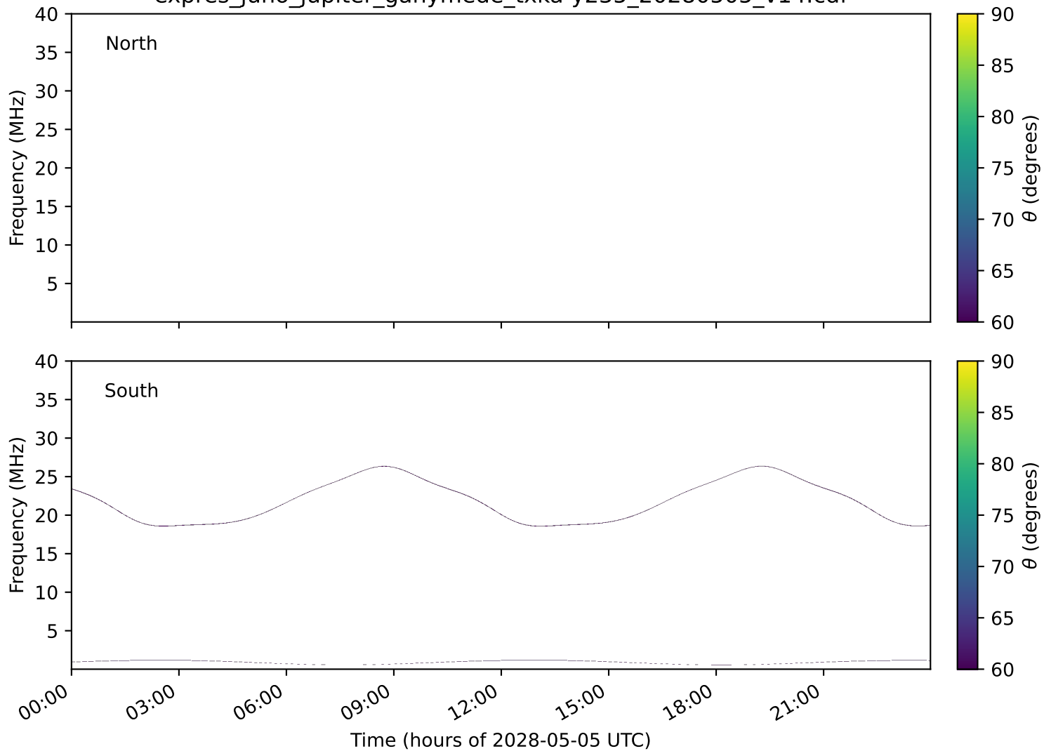
expres_juno_jupiter_ganymede_txka-y235_20280505_v14.cdf
