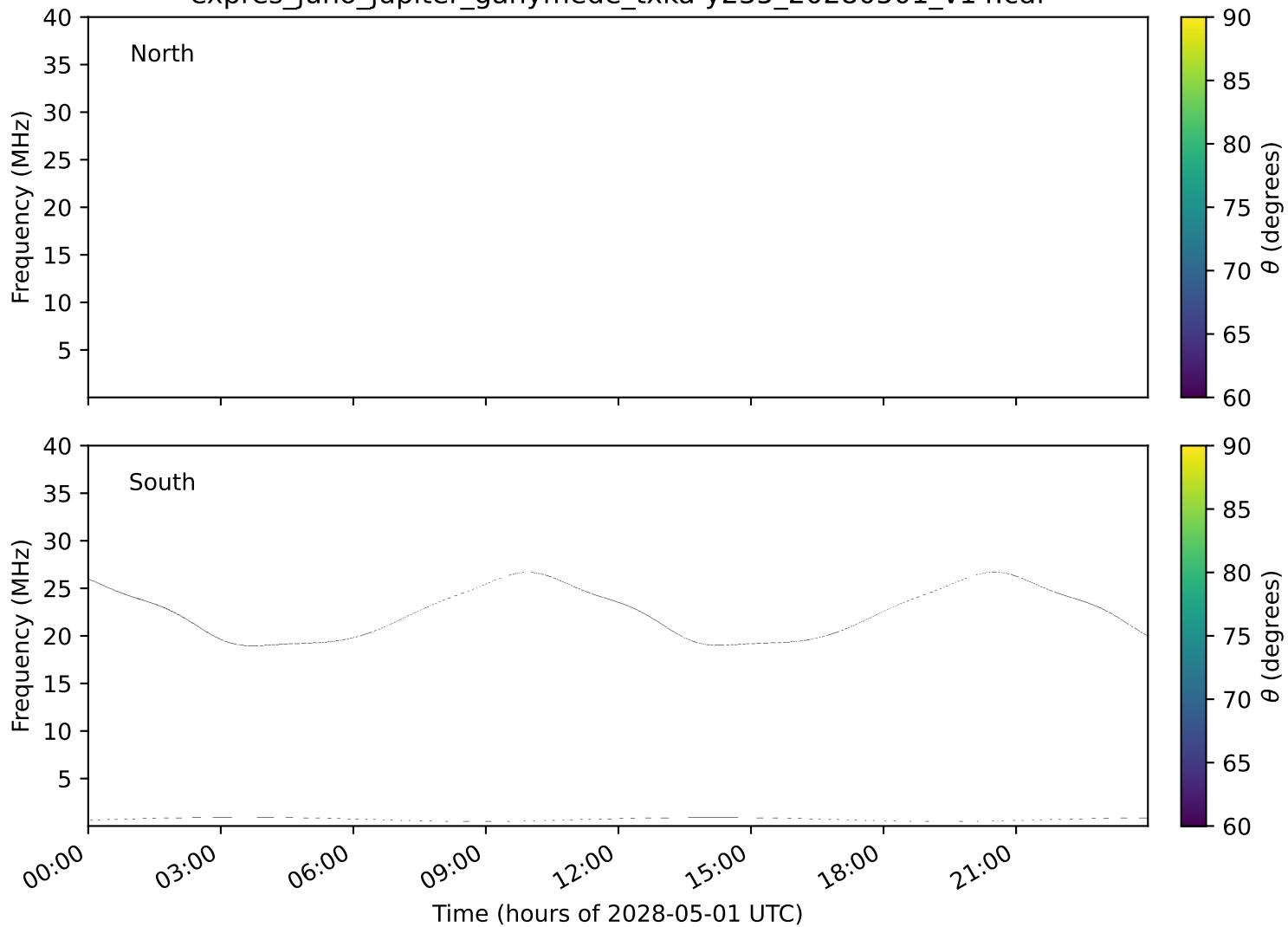
expres_juno_jupiter_ganymede_txka-y235_20280501_v14.cdf
