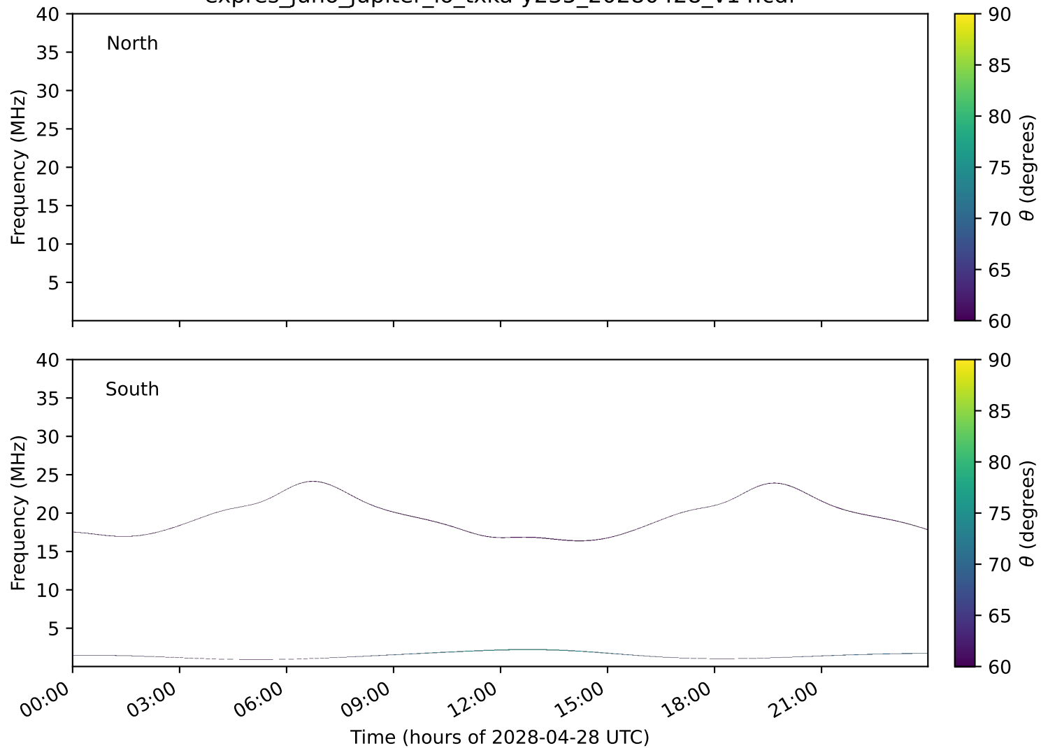
expres_juno_jupiter_io_txka-y235_20280428_v14.cdf
