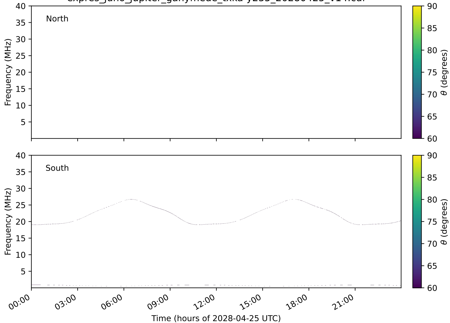
expres_juno_jupiter_ganymede_txka-y235_20280425_v14.cdf
