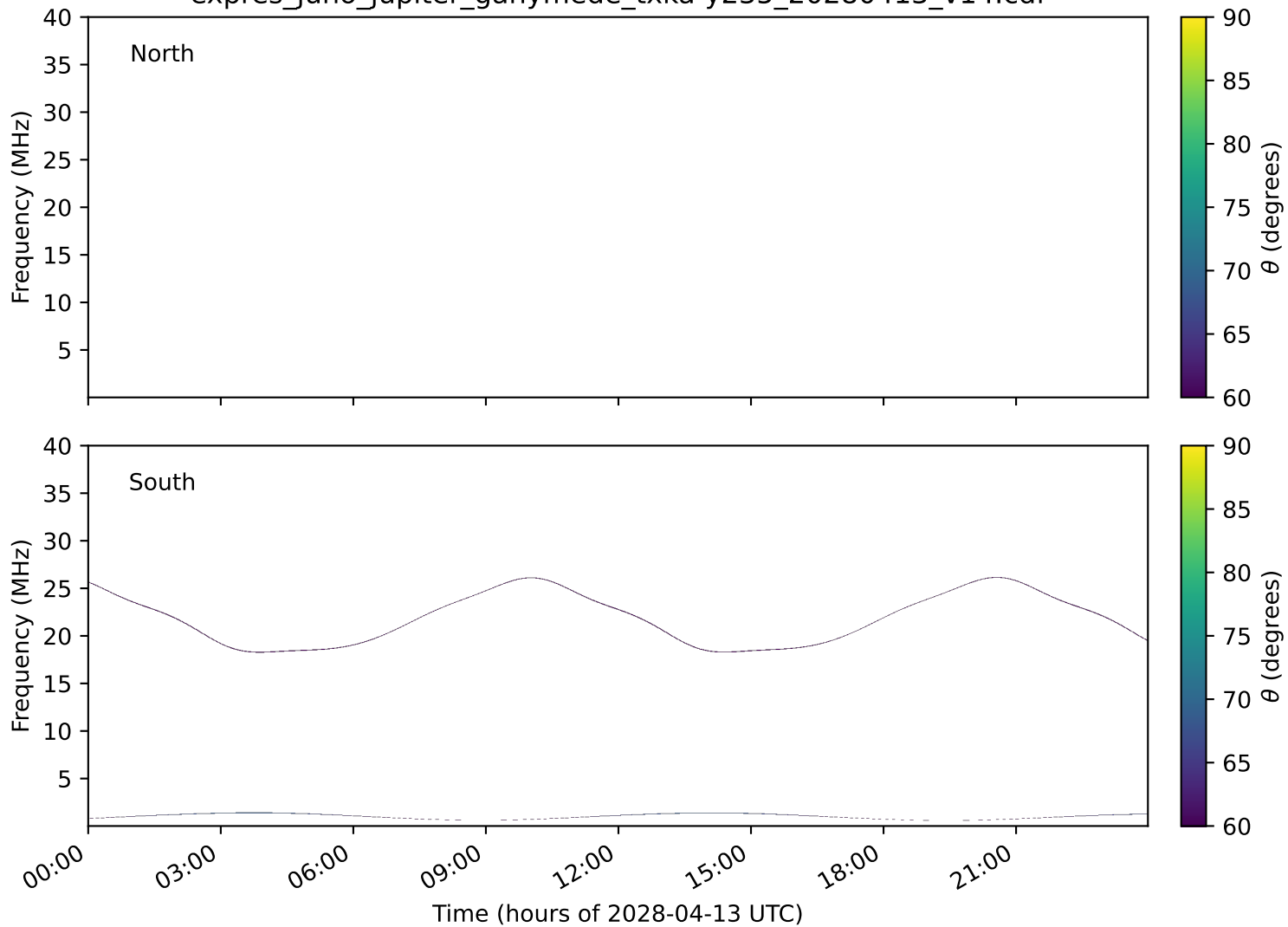
expres_juno_jupiter_ganymede_txka-y235_20280413_v14.cdf
