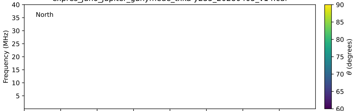
expres_juno_jupiter_ganymede_txka-y235_20280405_v14.cdf
