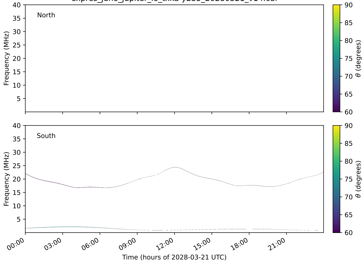
expres_juno_jupiter_io_txka-y235_20280321_v14.cdf
