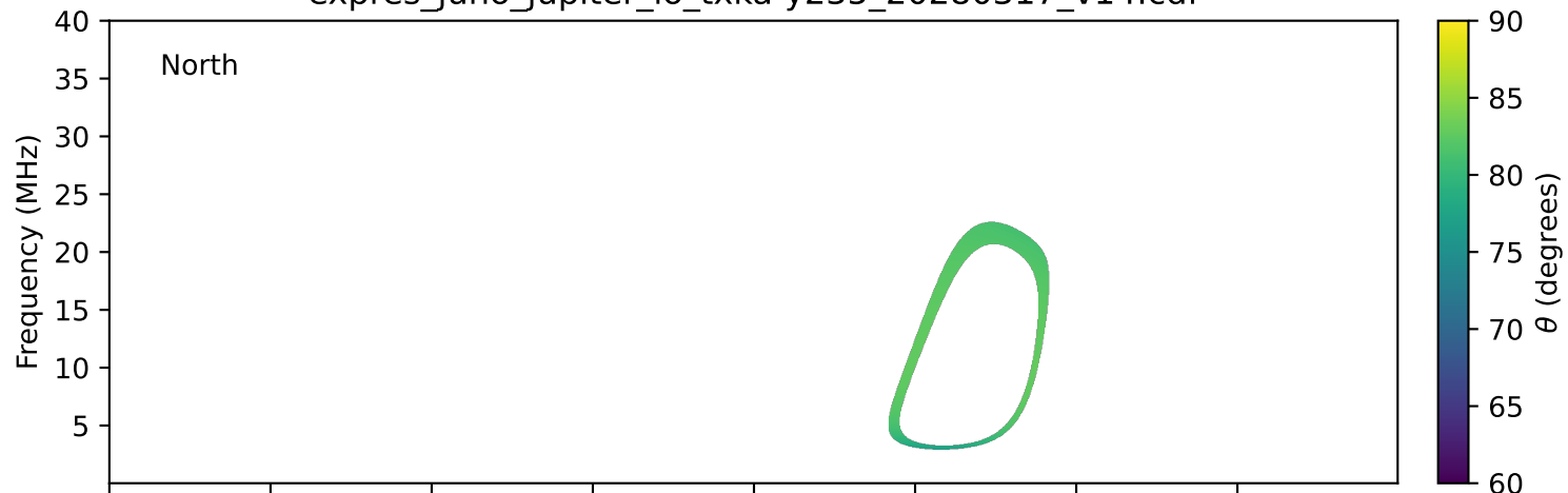
expres_juno_jupiter_io_txka-y235_20280317_v14.cdf
