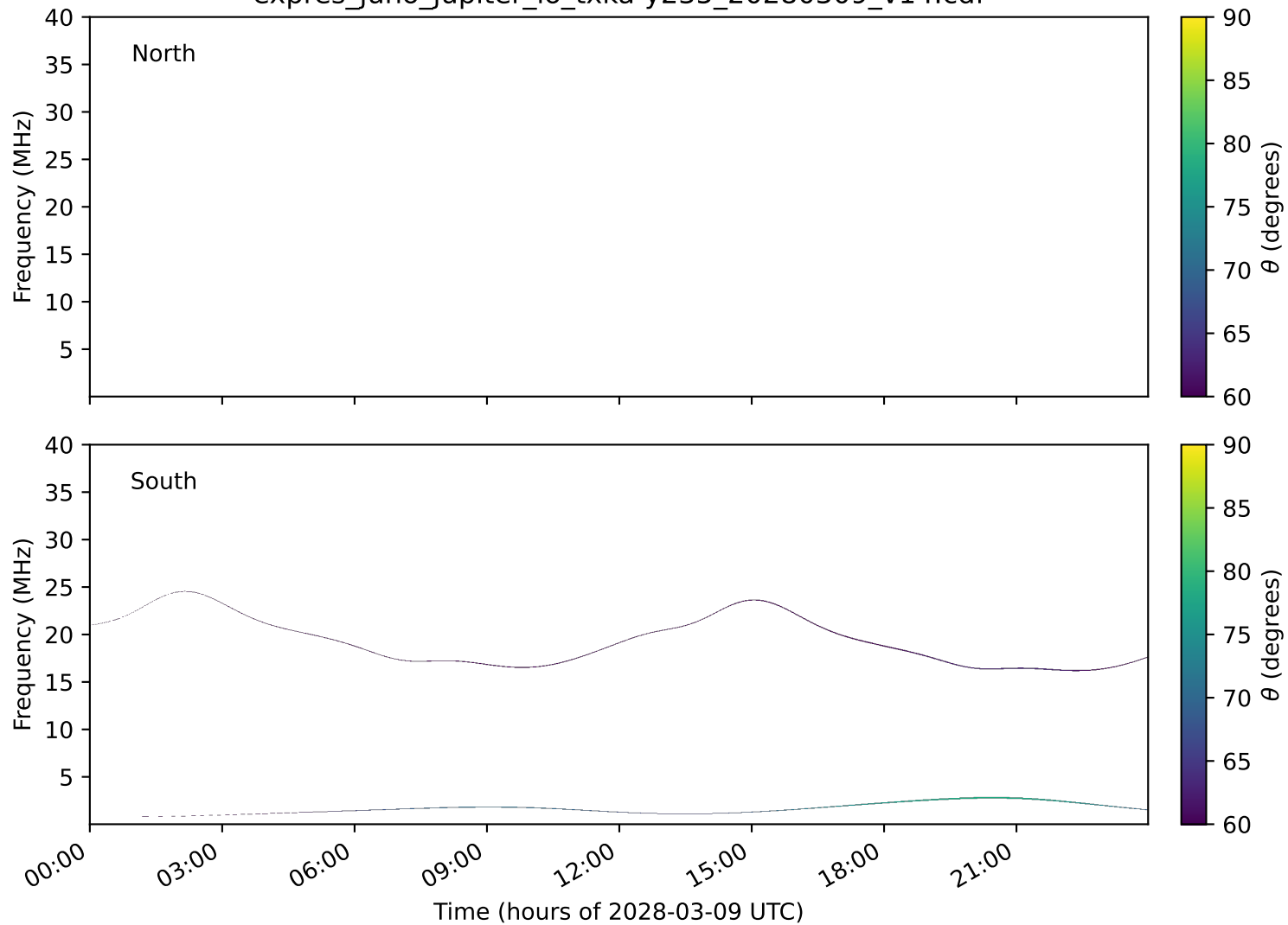
expres_juno_jupiter_io_txka-y235_20280309_v14.cdf
