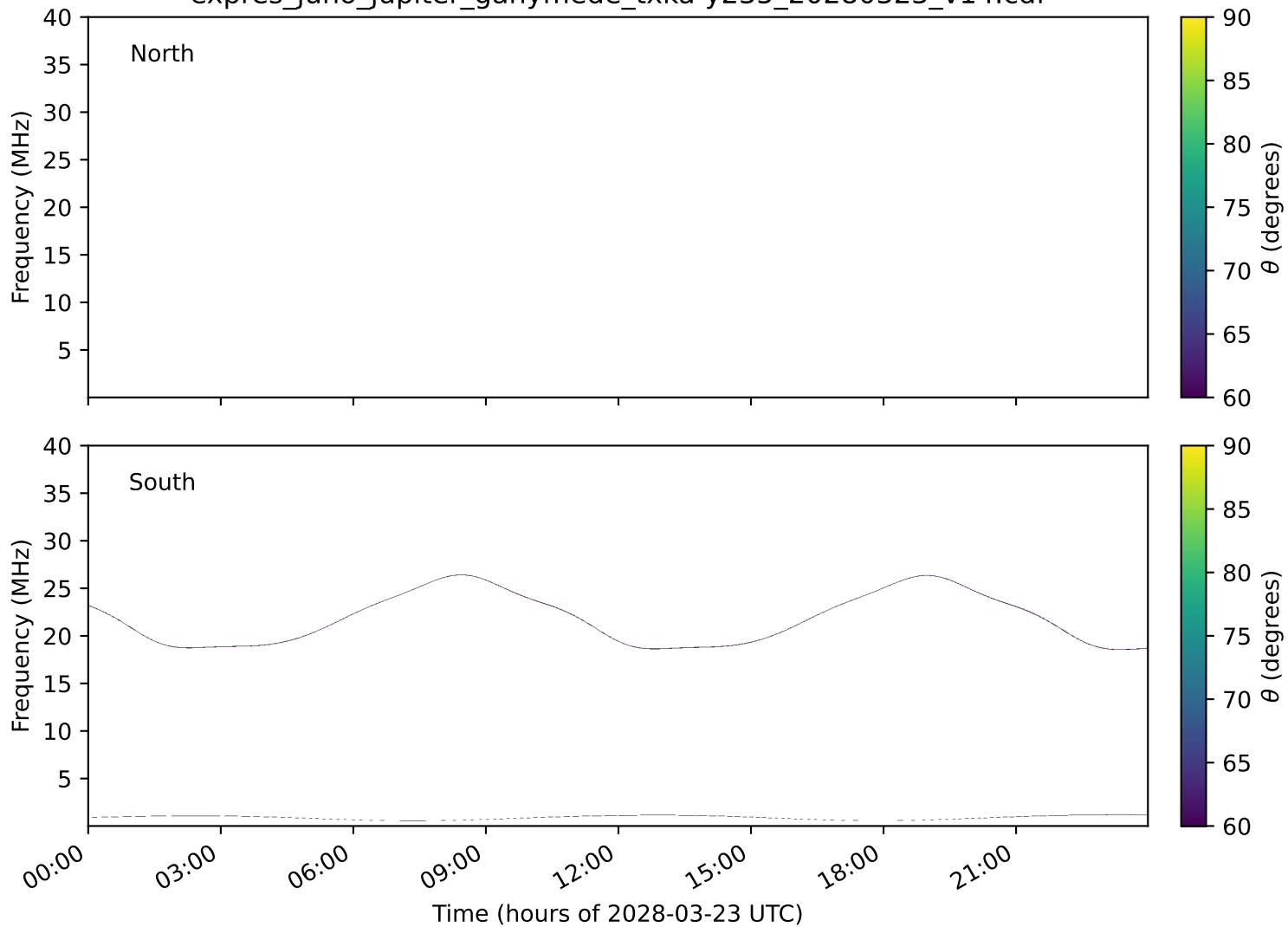
expres_juno_jupiter_ganymede_txka-y235_20280323_v14.cdf
