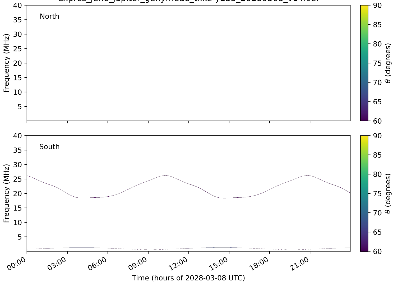
expres_juno_jupiter_ganymede_txka-y235_20280308_v14.cdf
