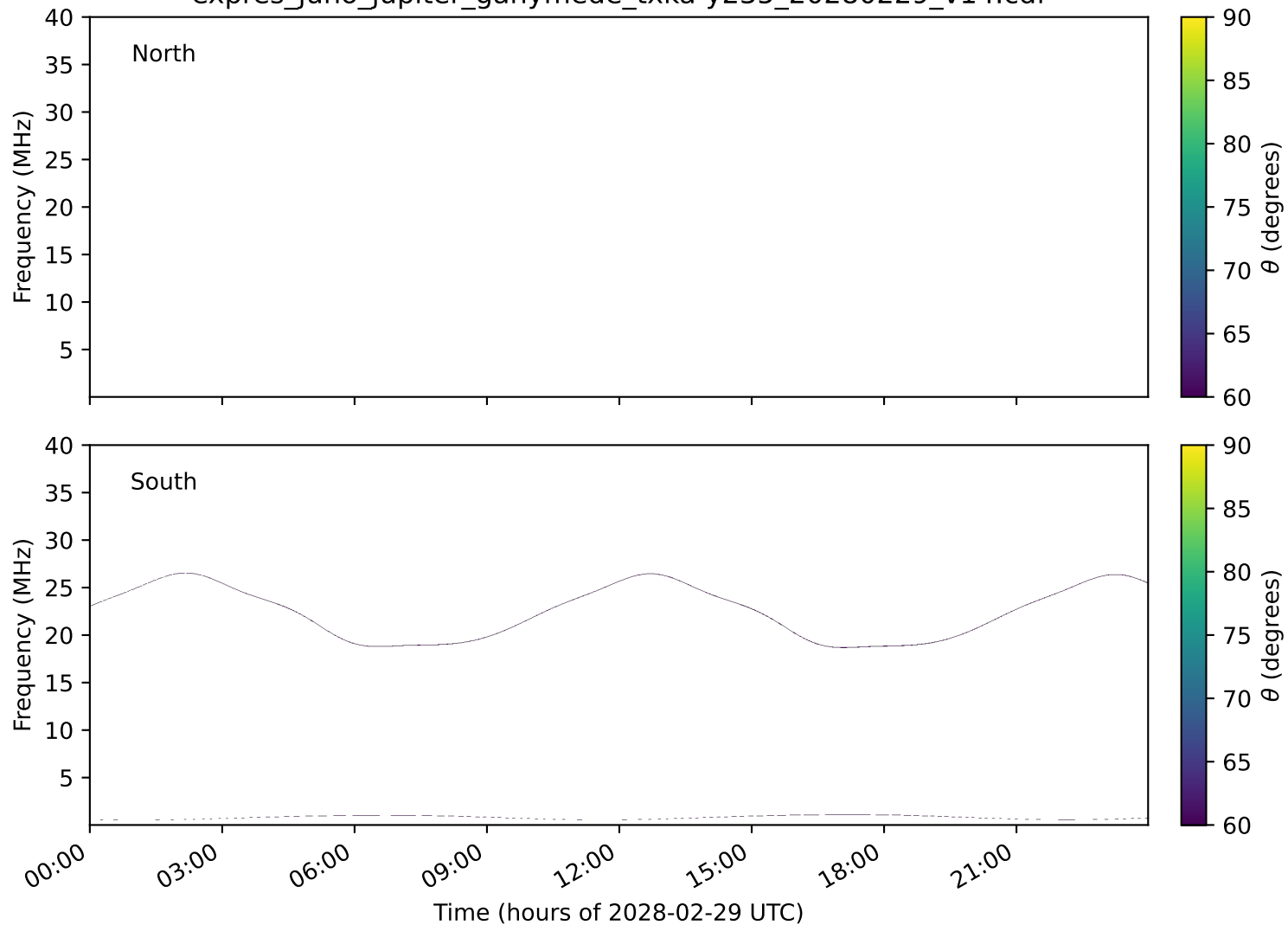
expres_juno_jupiter_ganymede_txka-y235_20280229_v14.cdf
