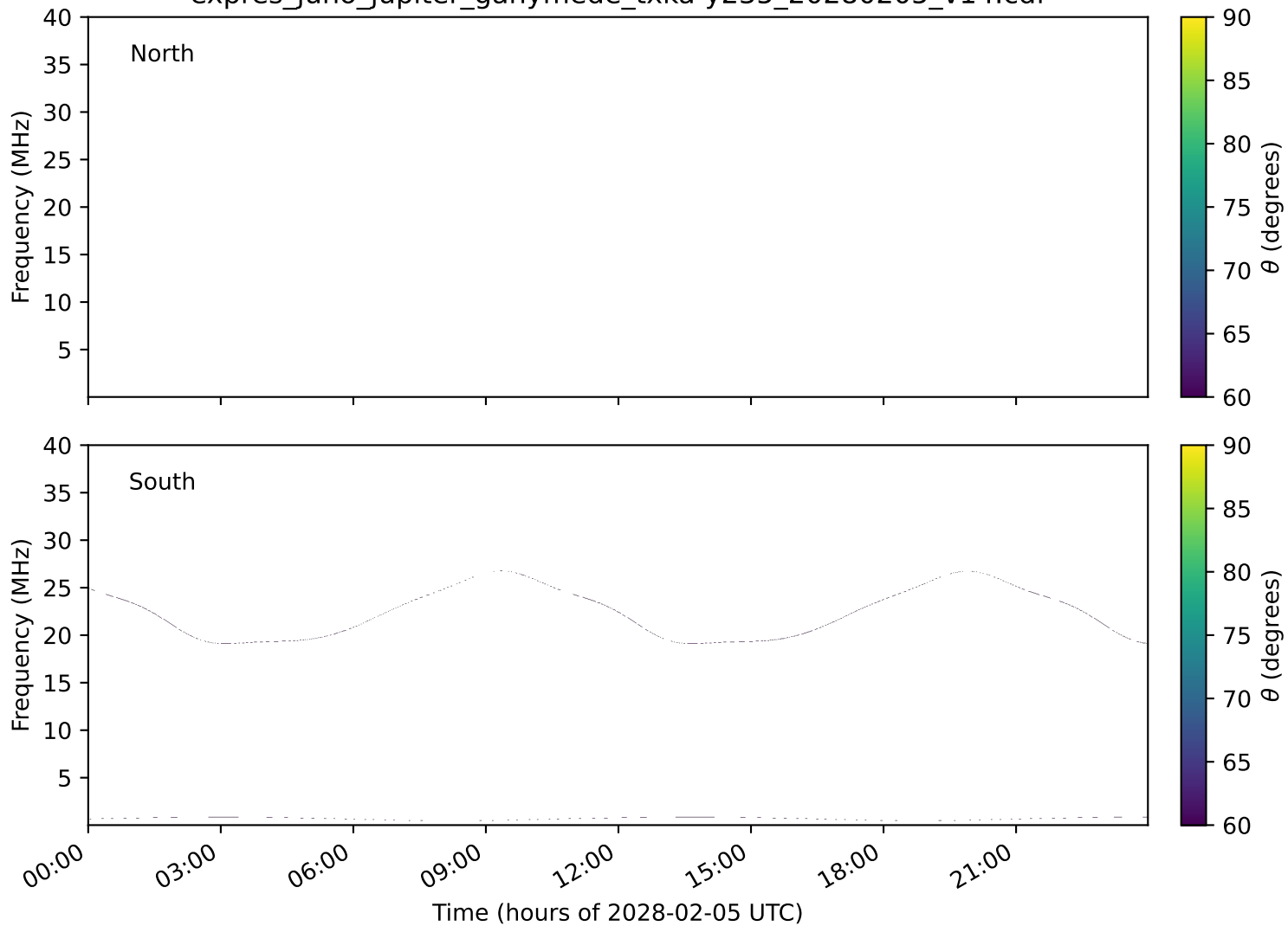
expres_juno_jupiter_ganymede_txka-y235_20280205_v14.cdf
