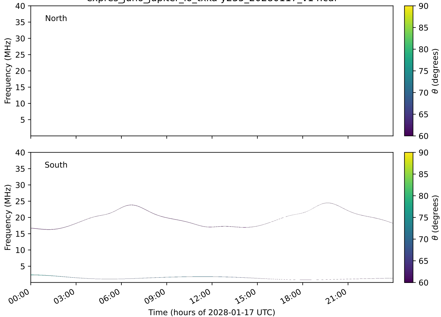
expres_juno_jupiter_io_txka-y235_20280117_v14.cdf
