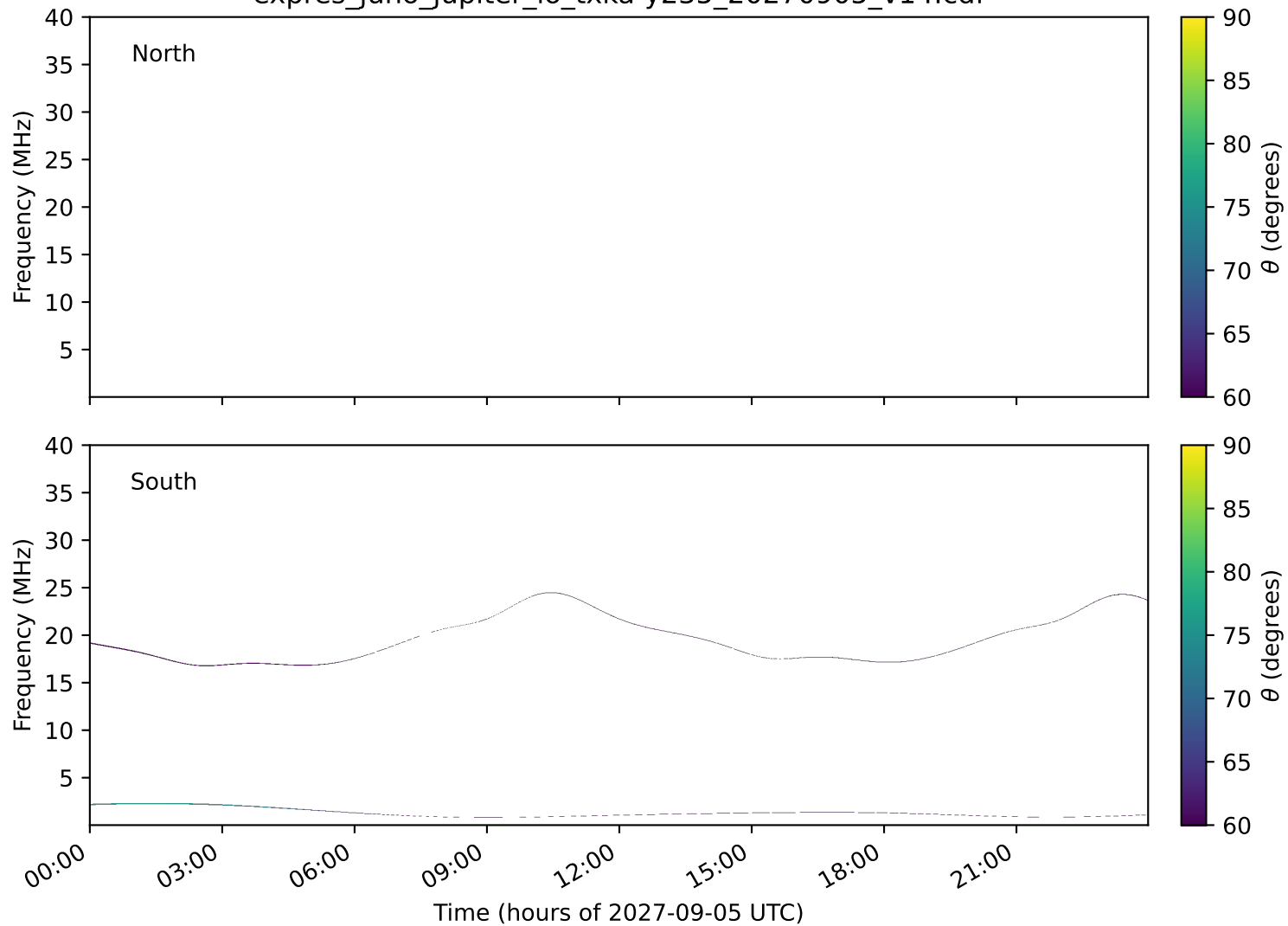
expres_juno_jupiter_io_txka-y235_20270905_v14.cdf
