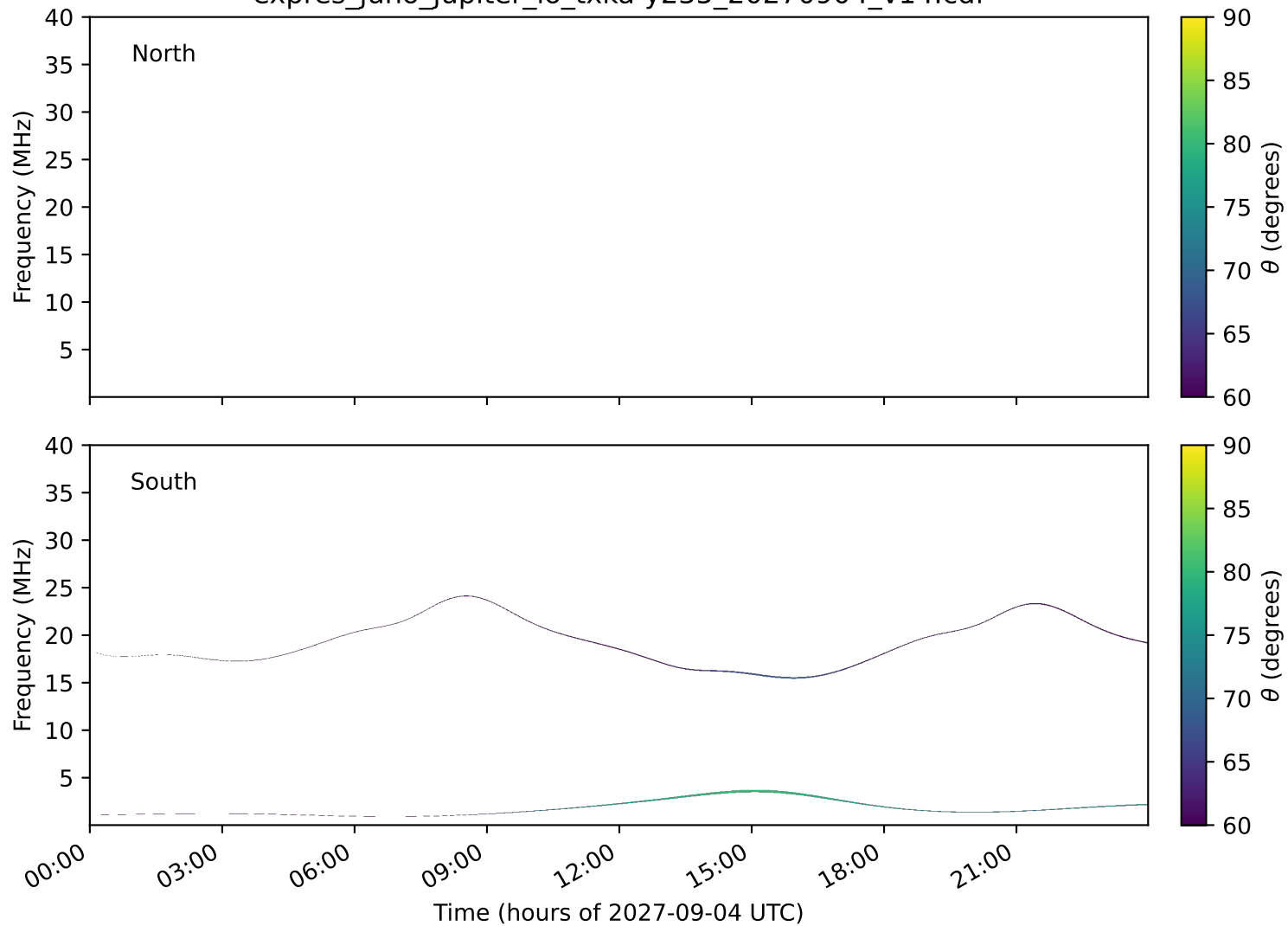
expres_juno_jupiter_io_txka-y235_20270904_v14.cdf
