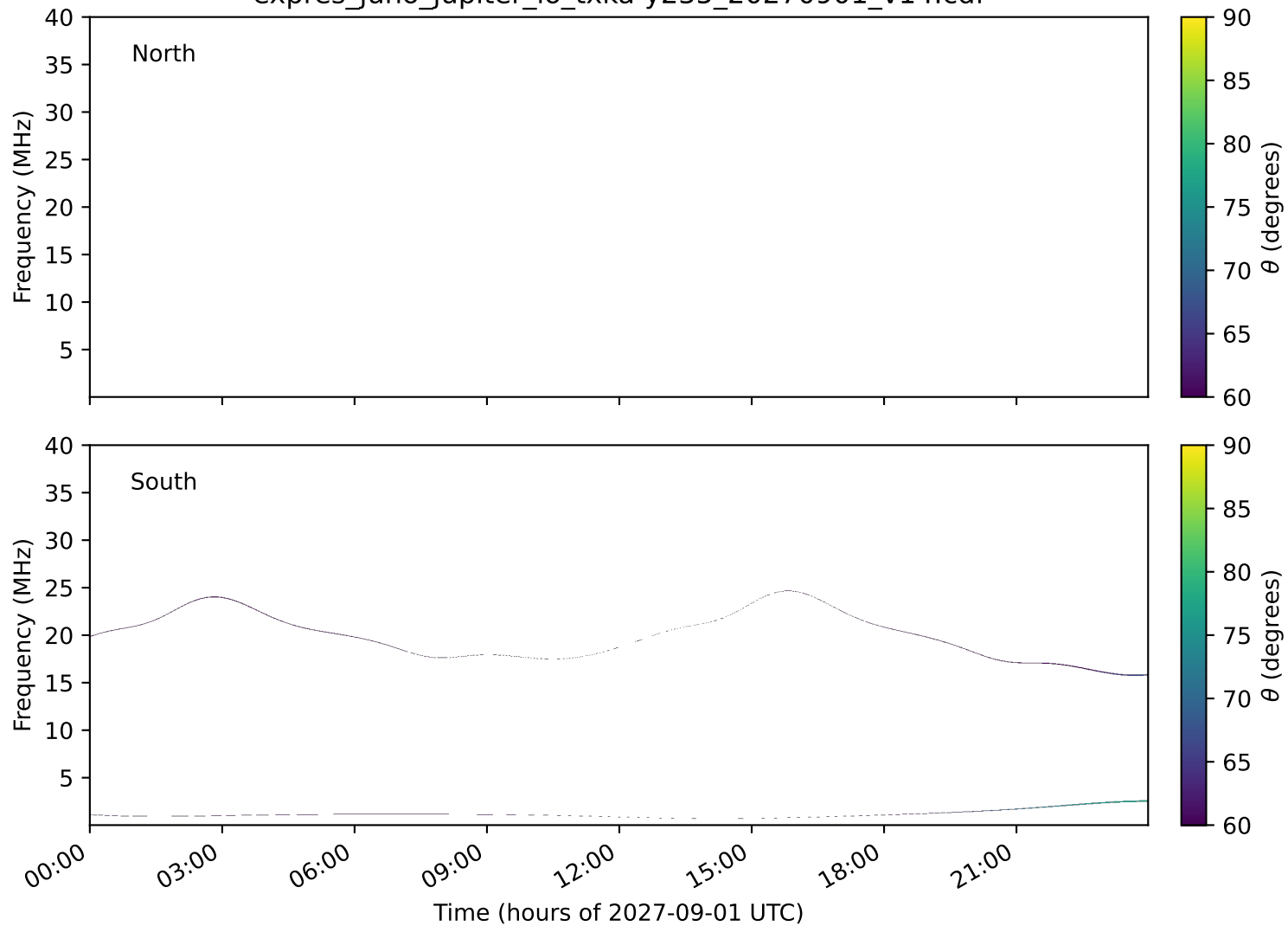
expres_juno_jupiter_io_txka-y235_20270901_v14.cdf
