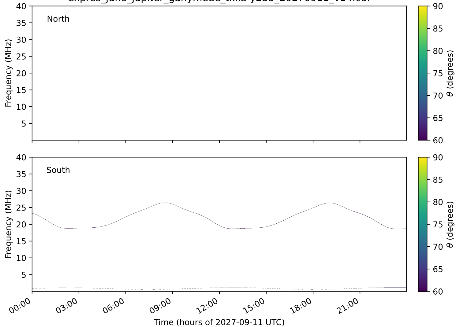
expres_juno_jupiter_ganymede_txka-y235_20270911_v14.cdf
