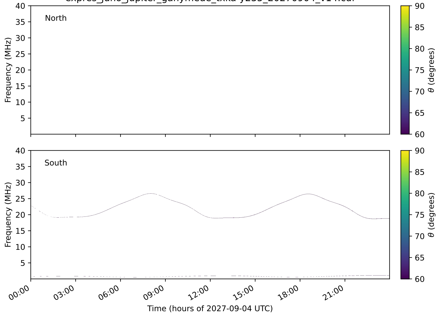
expres_juno_jupiter_ganymede_txka-y235_20270904_v14.cdf
