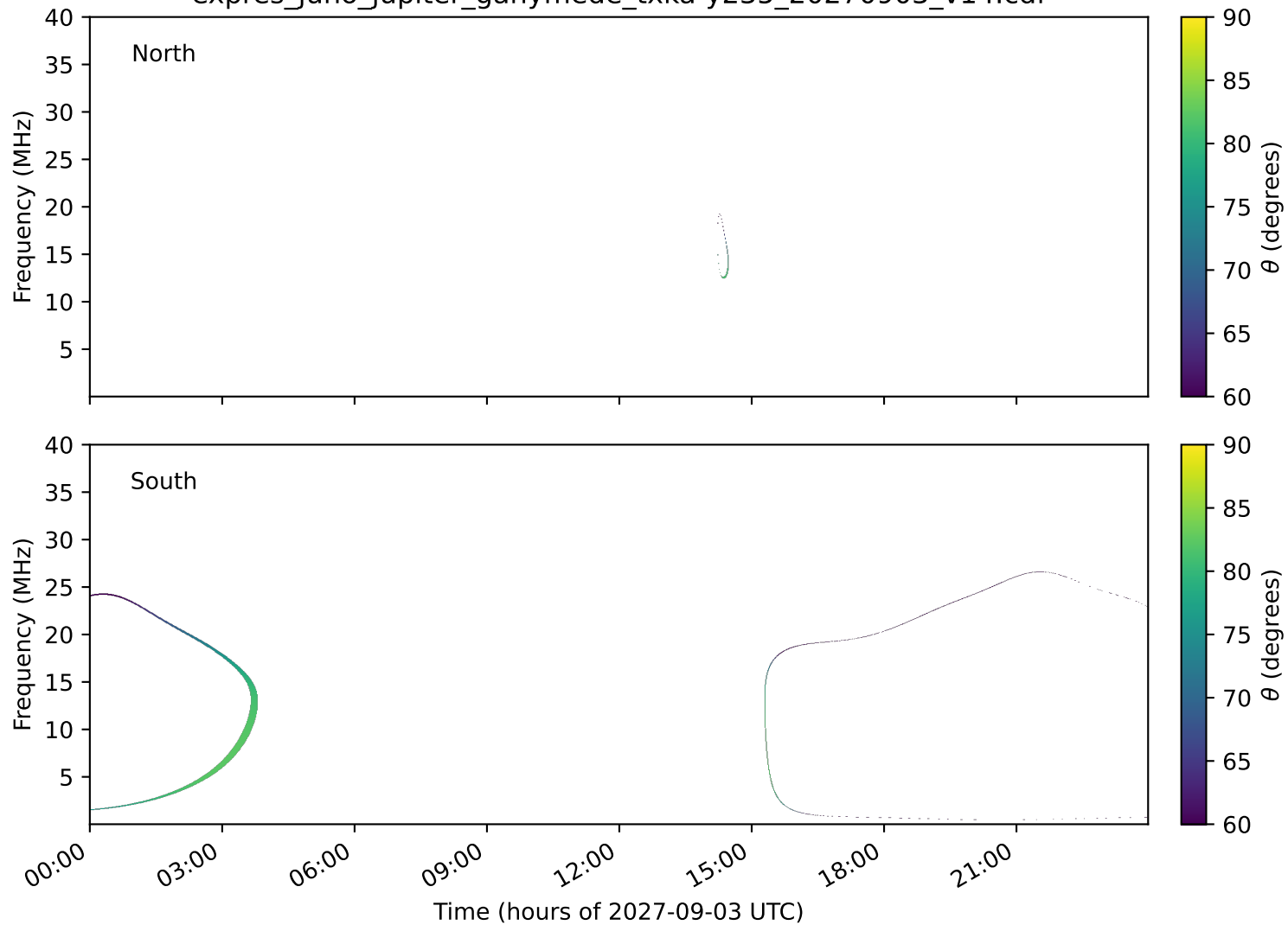
expres_juno_jupiter_ganymede_txka-y235_20270903_v14.cdf
