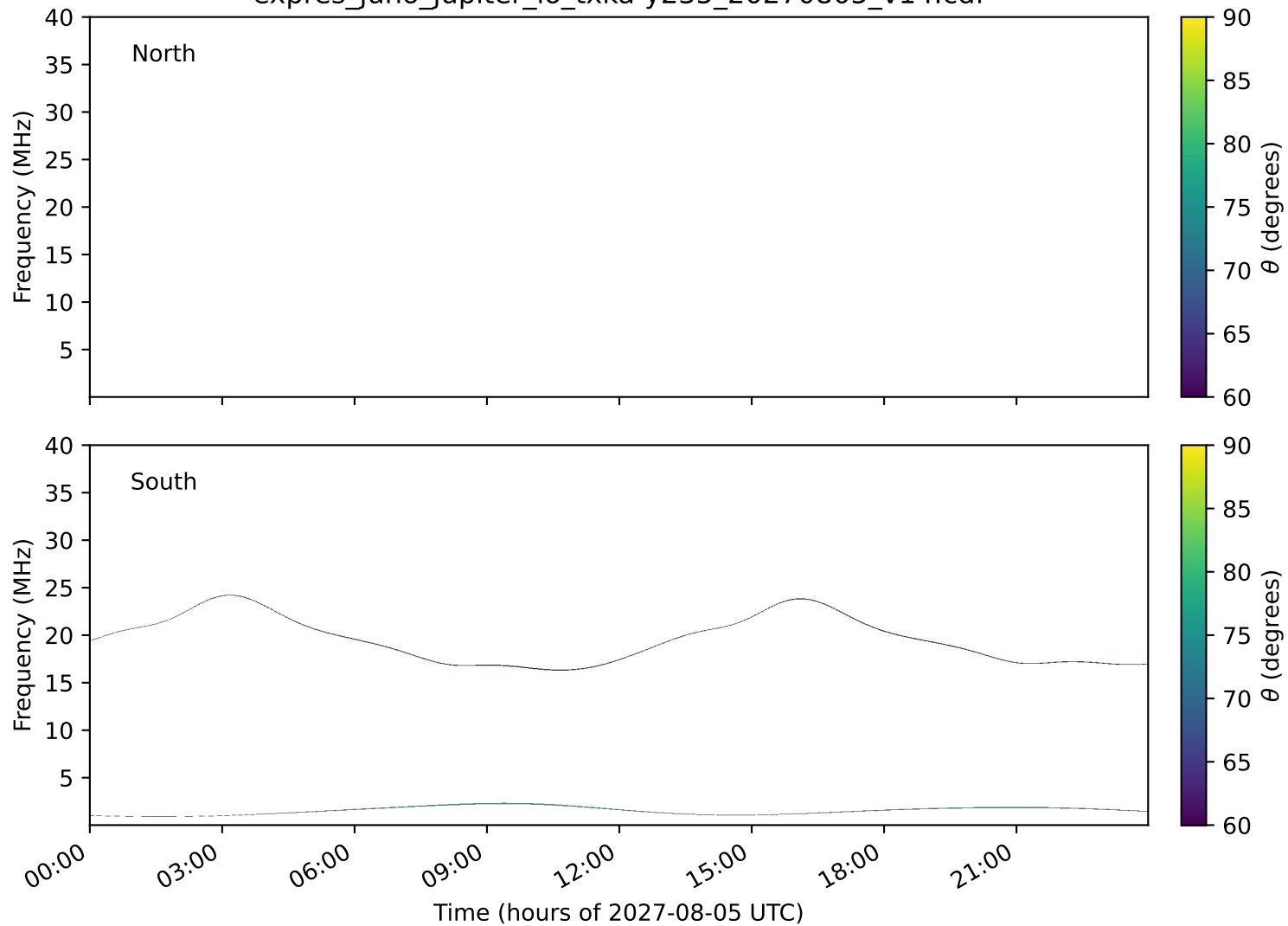
expres_juno_jupiter_io_txka-y235_20270805_v14.cdf
