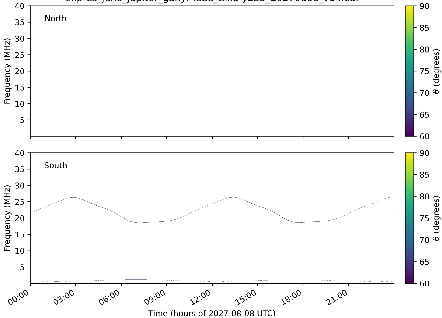
expres_juno_jupiter_ganymede_txka-y235_20270808_v14.cdf
