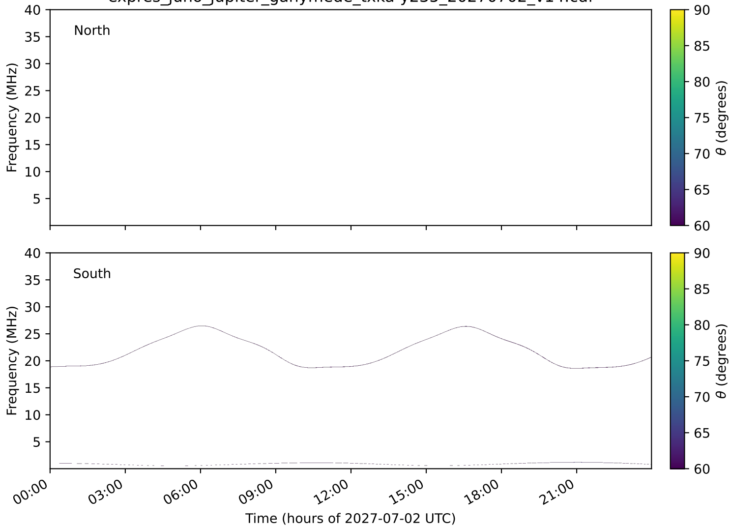
expres_juno_jupiter_ganymede_txka-y235_20270702_v14.cdf
