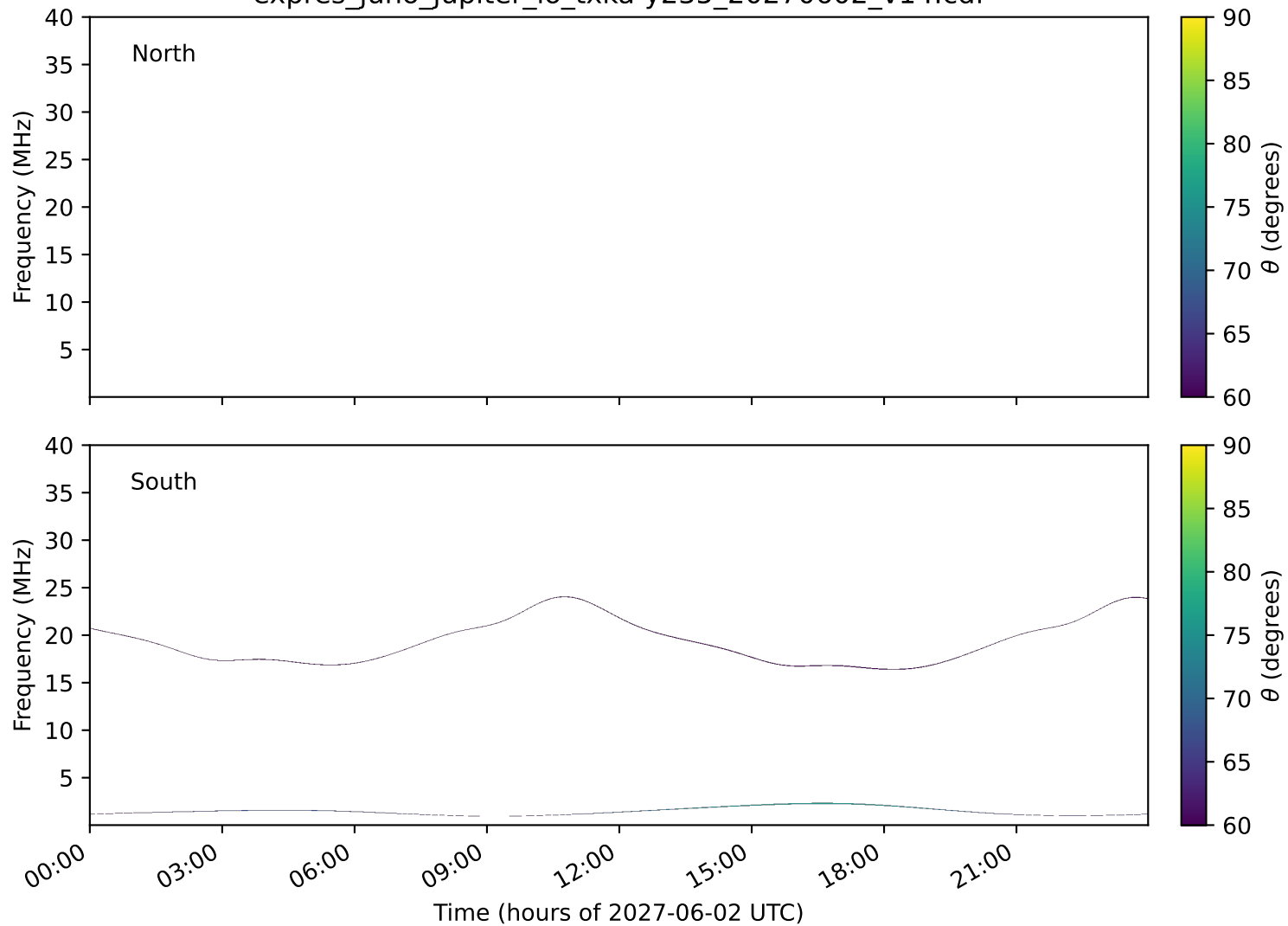
expres_juno_jupiter_io_txka-y235_20270602_v14.cdf
