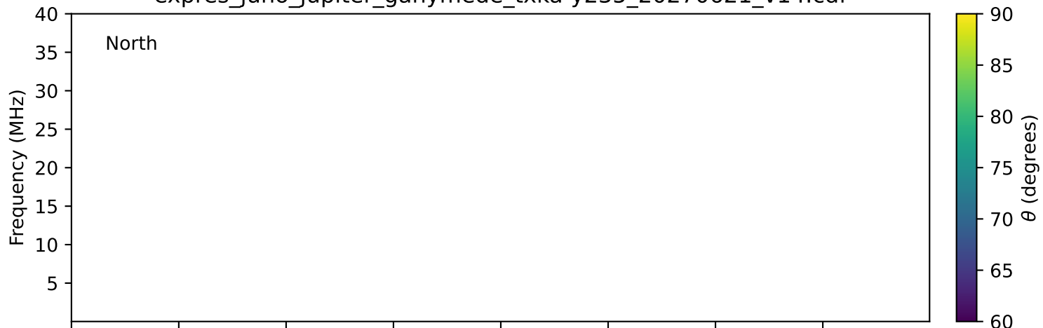
expres_juno_jupiter_ganymede_txka-y235_20270621_v14.cdf
