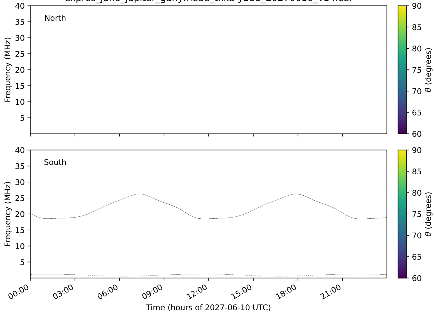
expres_juno_jupiter_ganymede_txka-y235_20270610_v14.cdf
