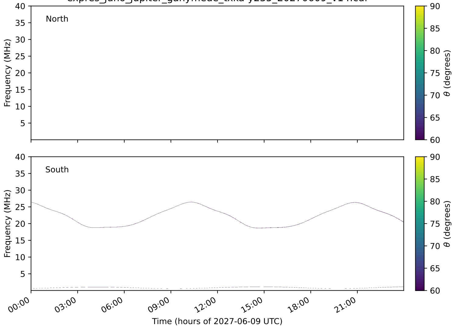
expres_juno_jupiter_ganymede_txka-y235_20270609_v14.cdf
