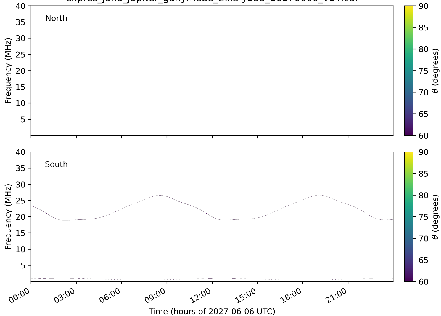
expres_juno_jupiter_ganymede_txka-y235_20270606_v14.cdf
