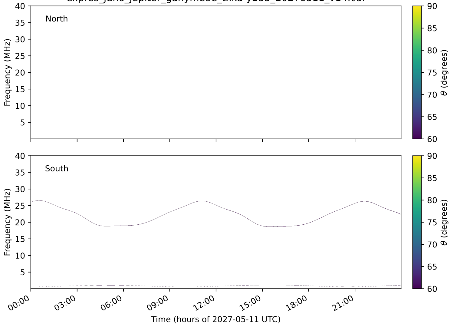
expres_juno_jupiter_ganymede_txka-y235_20270511_v14.cdf
