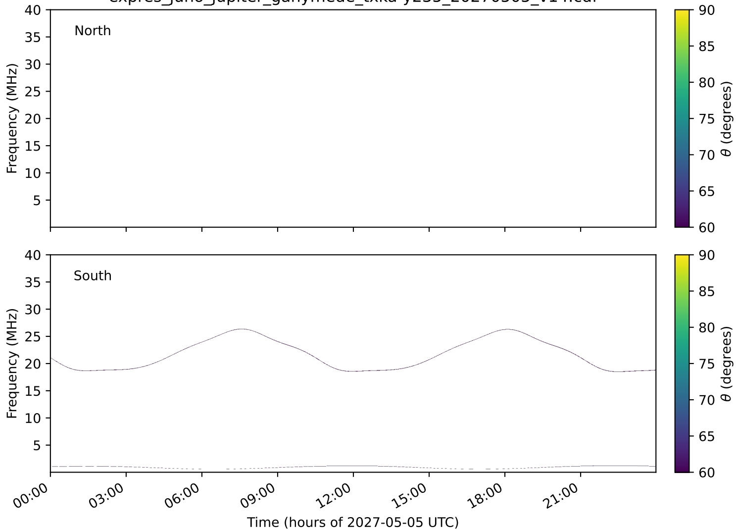
expres_juno_jupiter_ganymede_txka-y235_20270505_v14.cdf
