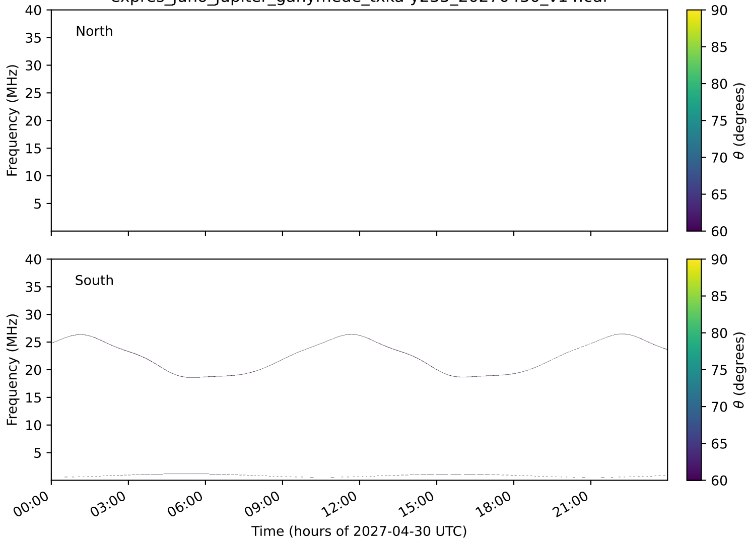
expres_juno_jupiter_ganymede_txka-y235_20270430_v14.cdf
