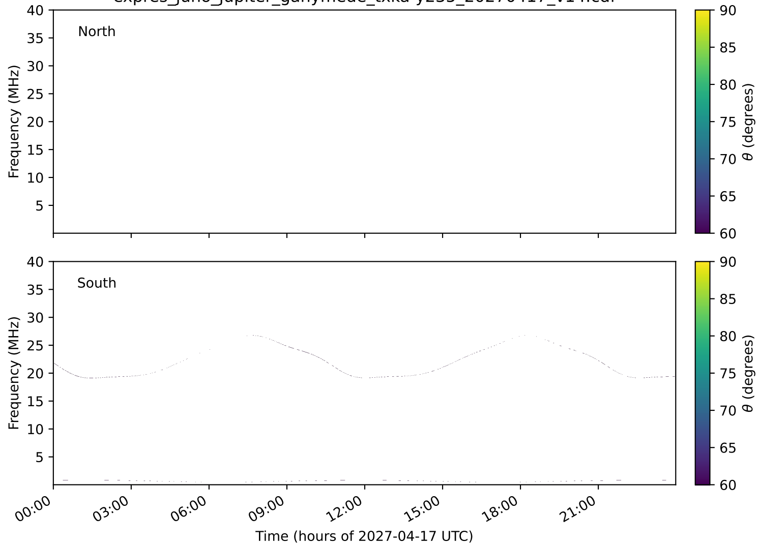
expres_juno_jupiter_ganymede_txka-y235_20270417_v14.cdf
