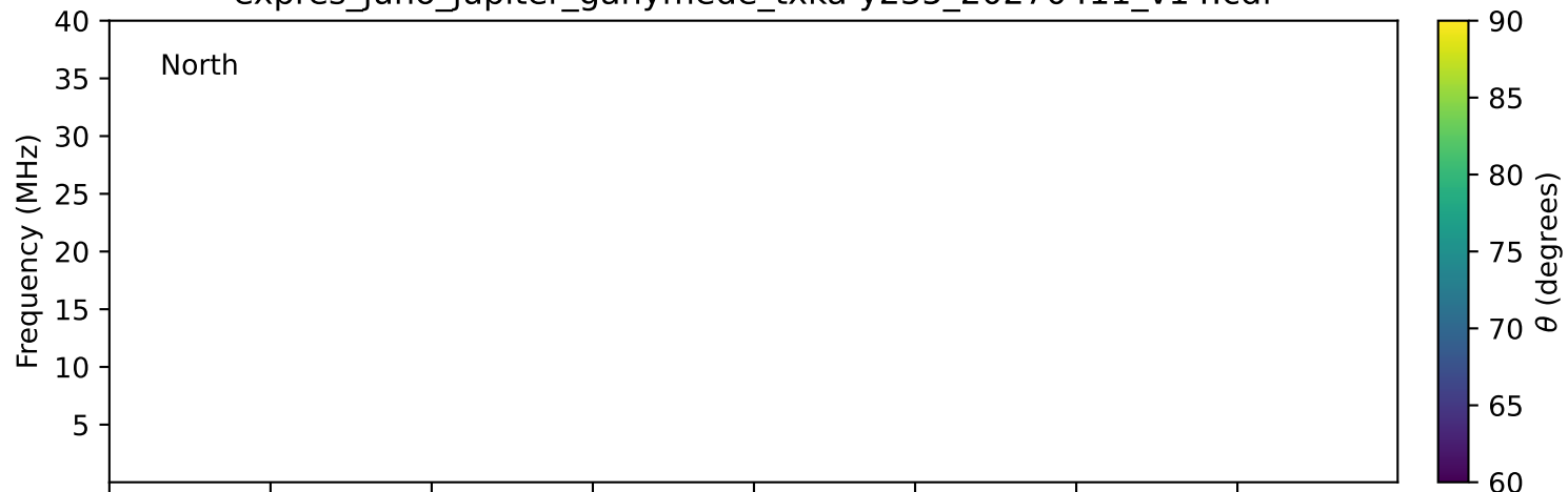
expres_juno_jupiter_ganymede_txka-y235_20270411_v14.cdf
