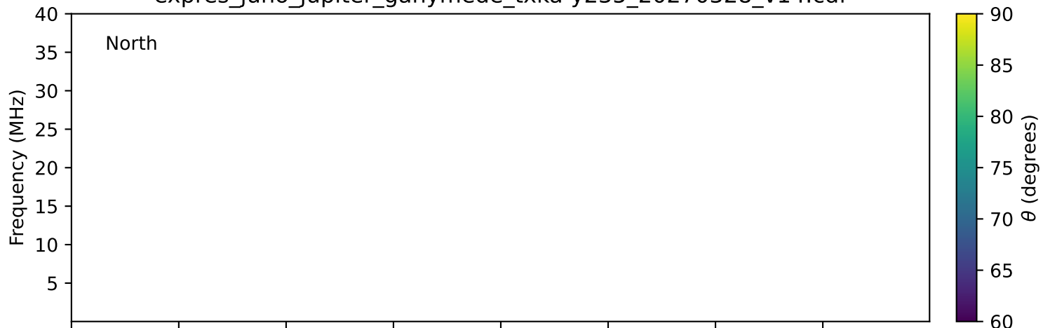
expres_juno_jupiter_ganymede_txka-y235_20270328_v14.cdf
