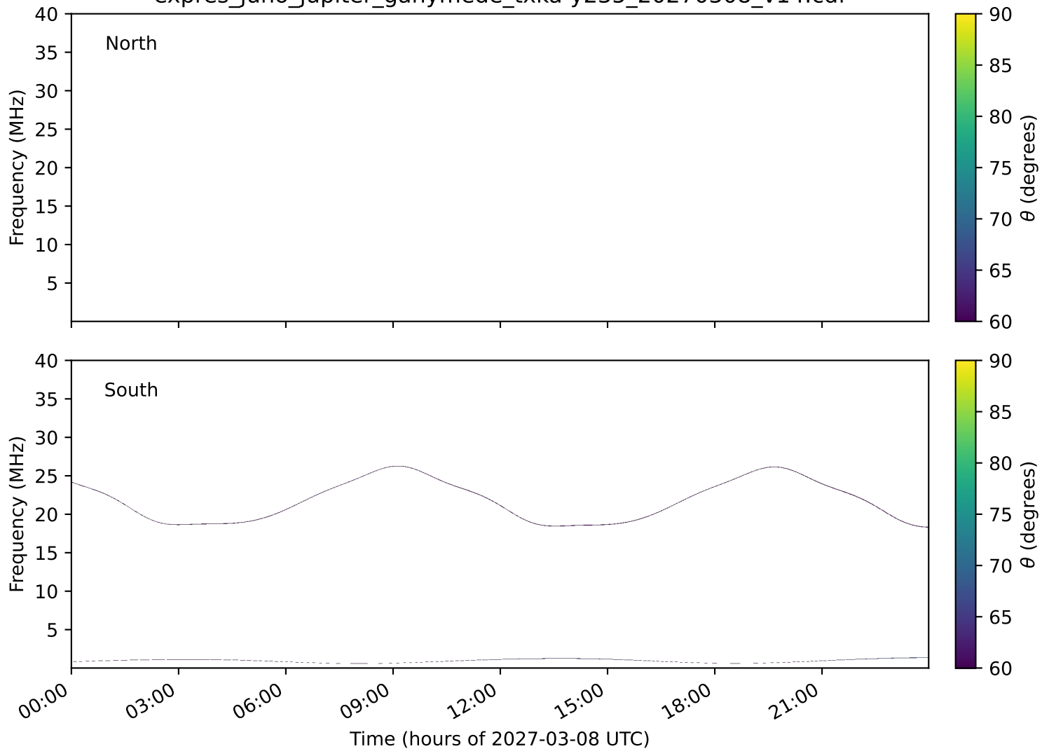
expres_juno_jupiter_ganymede_txka-y235_20270308_v14.cdf
