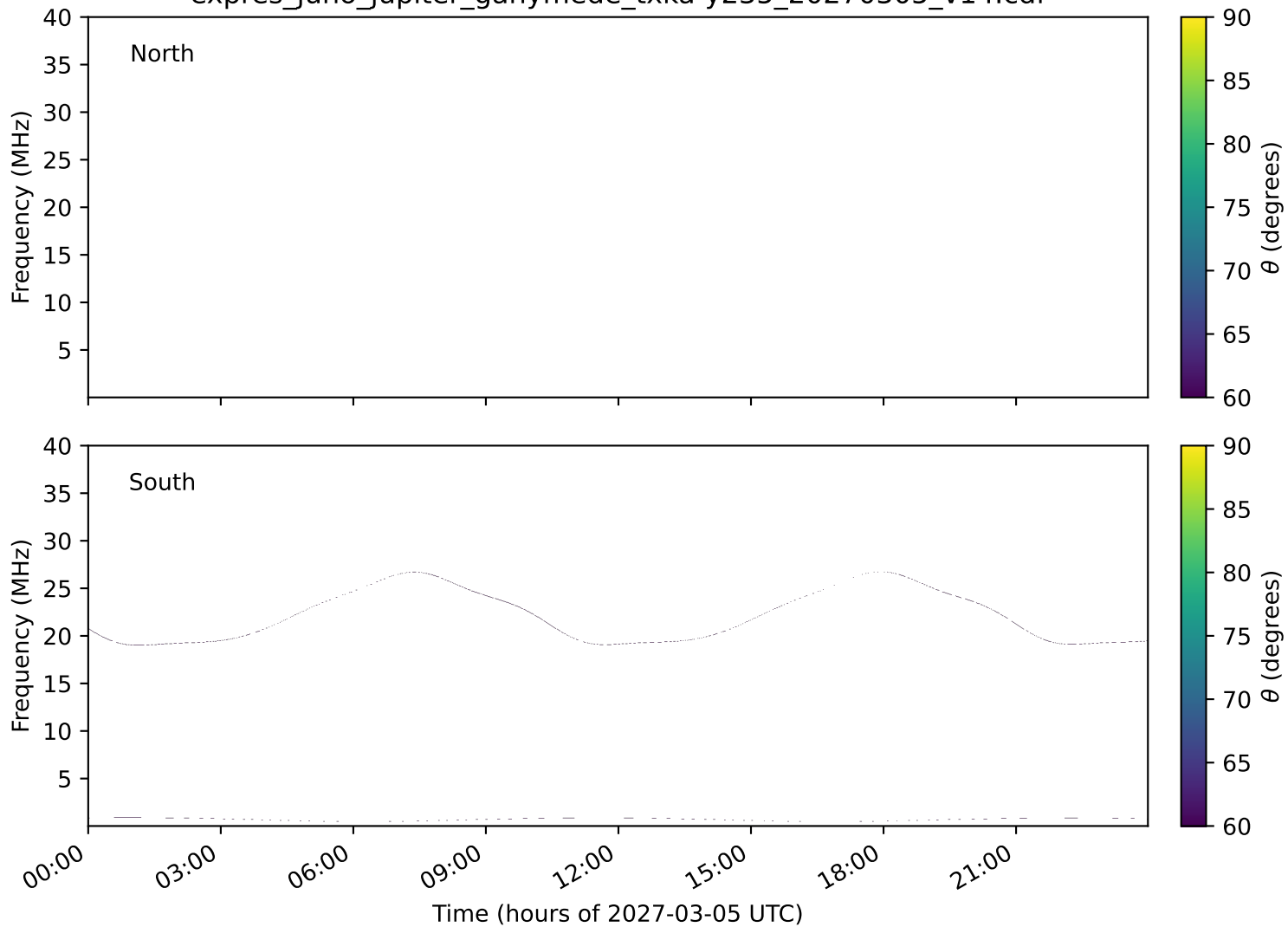
expres_juno_jupiter_ganymede_txka-y235_20270305_v14.cdf
